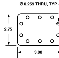
WR229 (UG-1727/U)
